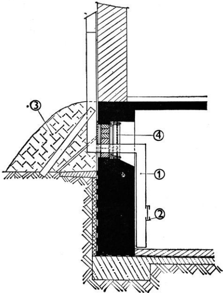
Obr. č. 7 Zhmotnenie okna pri inštalácii nasávacieho vzduchovodu, (1) nasávací vzduchovod, (2) regulovateľný uzáver prívodu vzduchu, (3) násyp zeminy, (4) tesniaca fólia.
